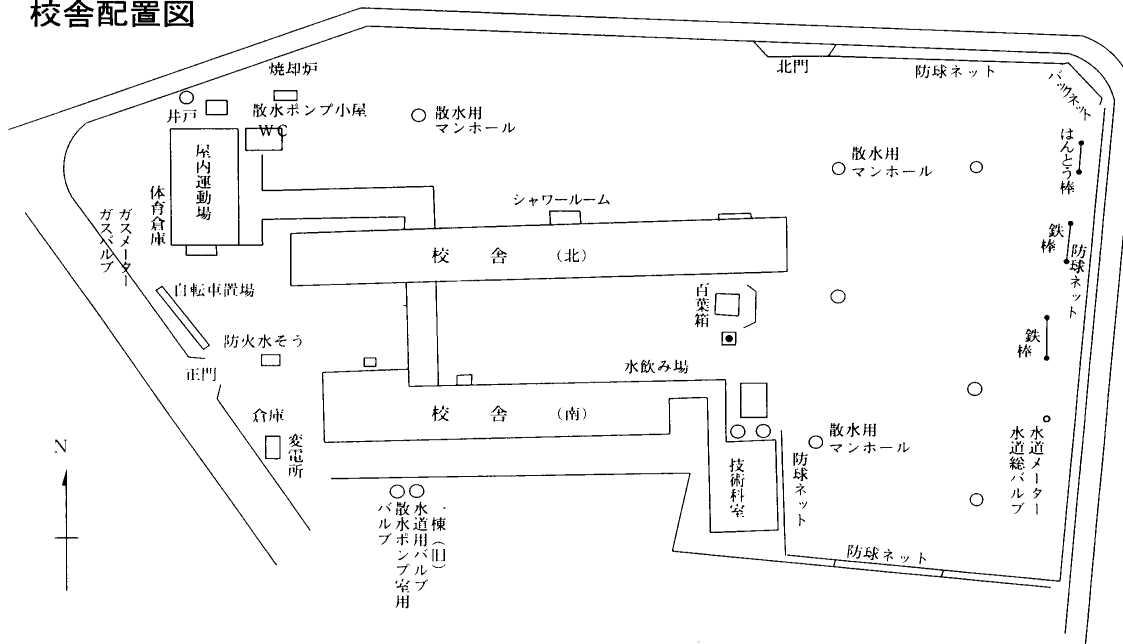
校舎配置図
